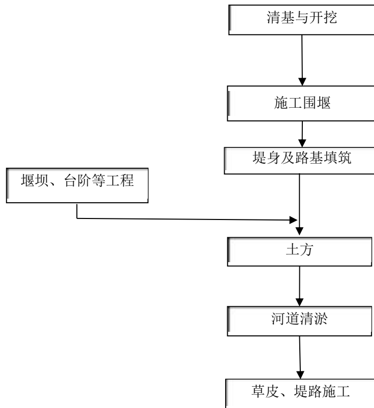
图 4-1 施工顺序图
