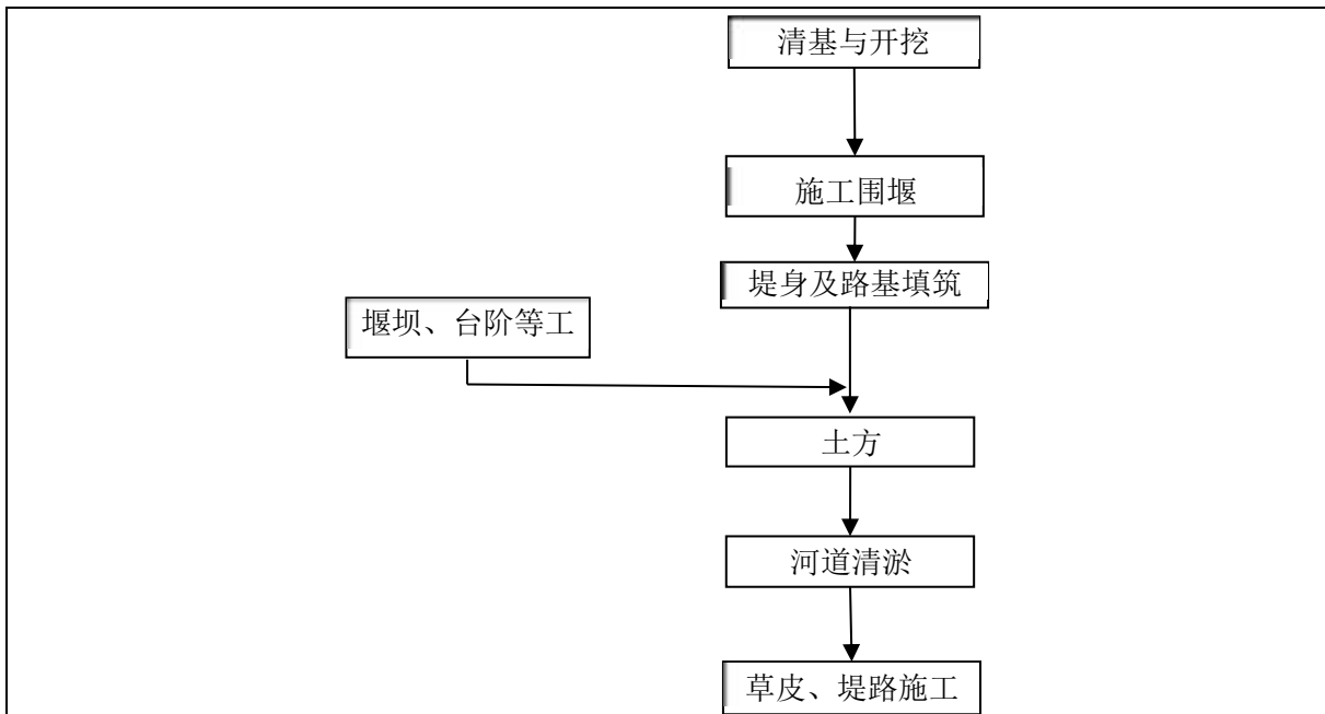
图 4-1 施工顺序图
