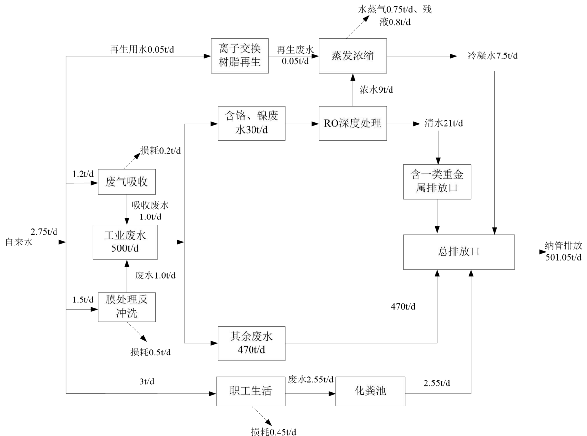
图 3.4-1 水平衡图
