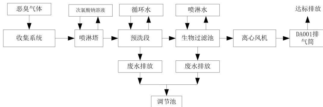
图 6.1-1 化学洗涤+生物除臭系统工艺流程
