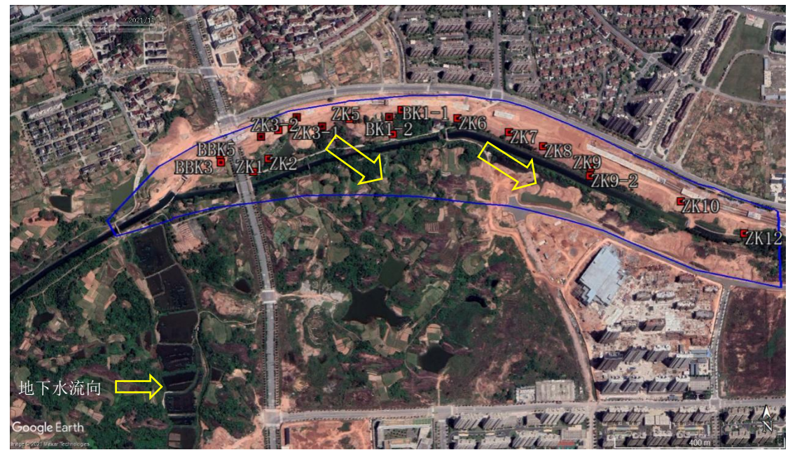
图 3-8 东港中心区段乌引干渠改线工程地下水勘测点位
