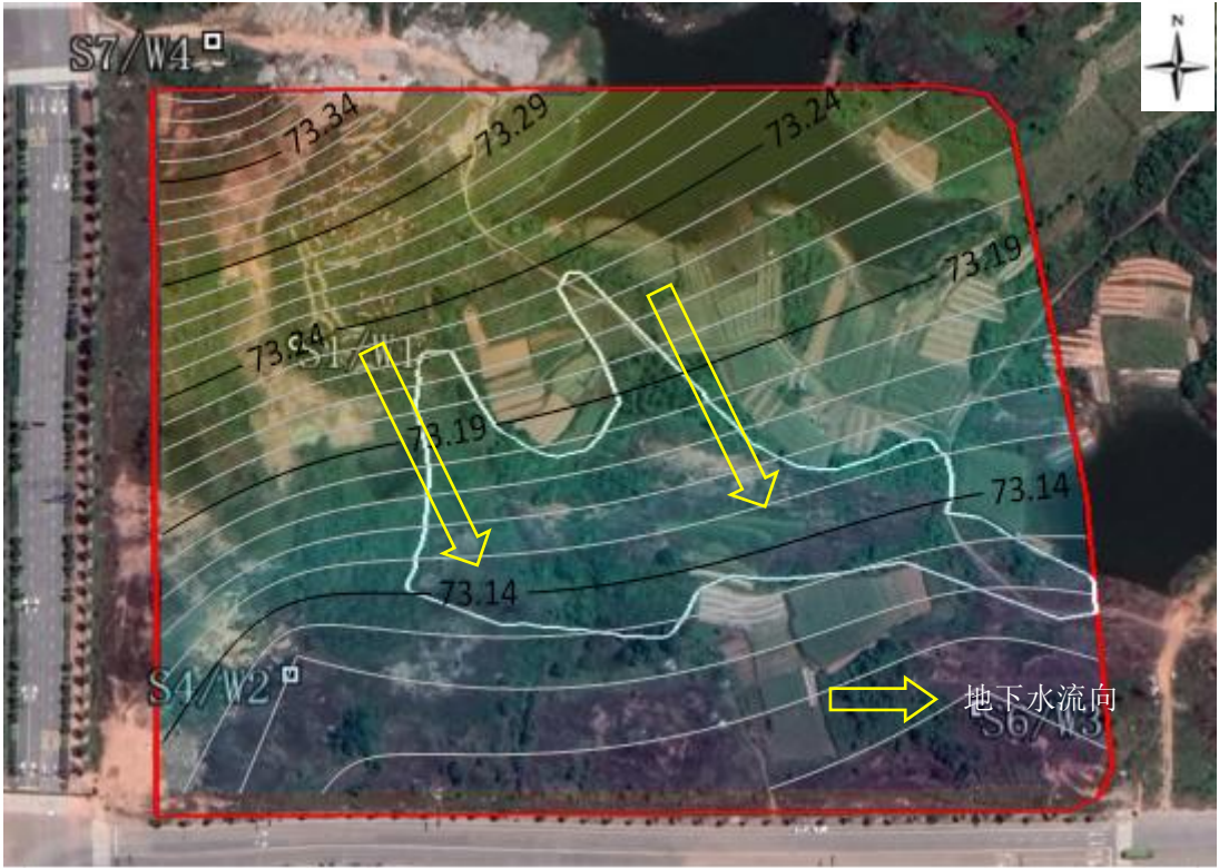
图 5-8 东港片区(中片)G-44#地块地下水流向图
